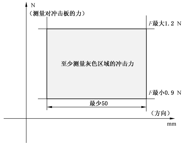
图 11 冲击力分布
